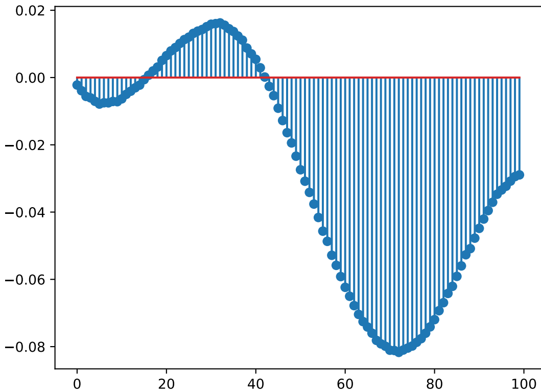
Vectorul de autocorelatie
