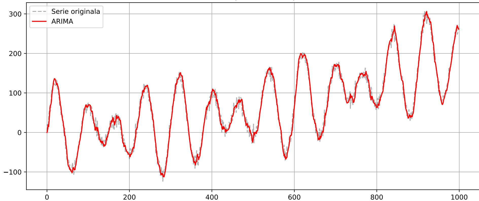
ARIMA cu p = 2 , d = 1 , q = 2
