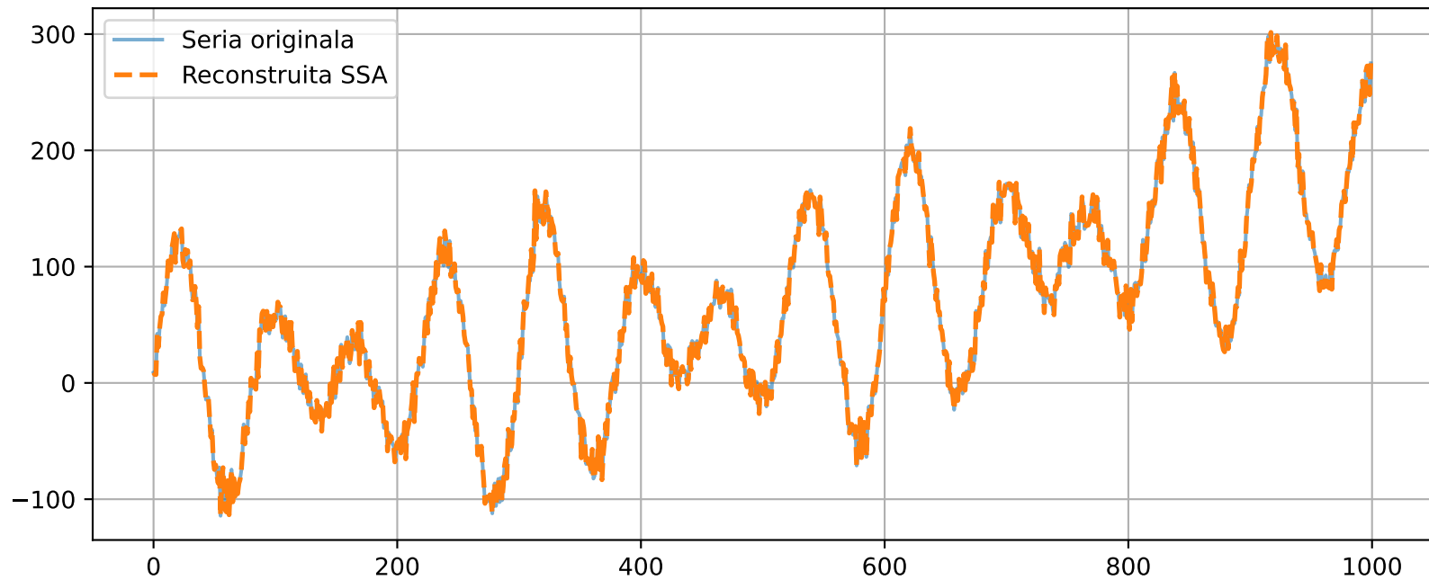
Reconstructia seriei prin SSA
