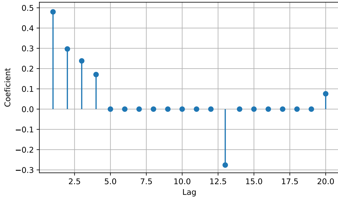
AR sparse - Greedy
