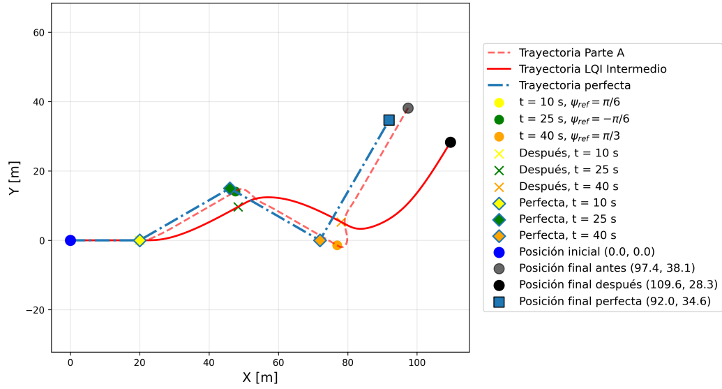
Figura 13: Comparación de trayectorias entre Parte A, LQI intermedio y trayectoria ideal.
