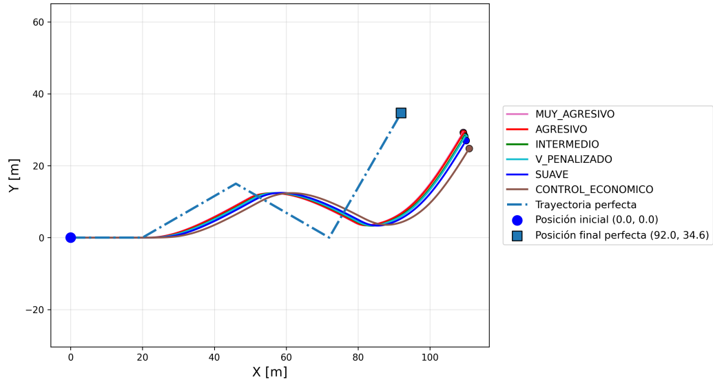
Figura 12: Trayectorias reconstruidas para los seis controladores LQI y trayectoria ideal.
