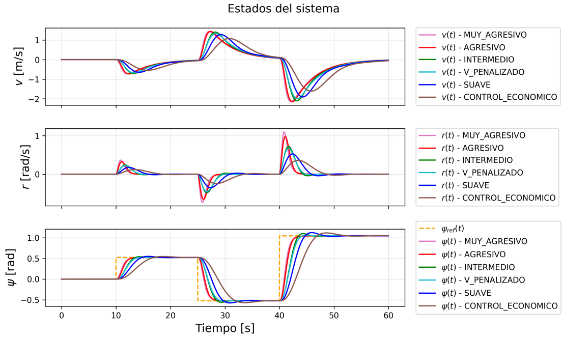
Figura 8: Estados del sistema para los casos LQI.
