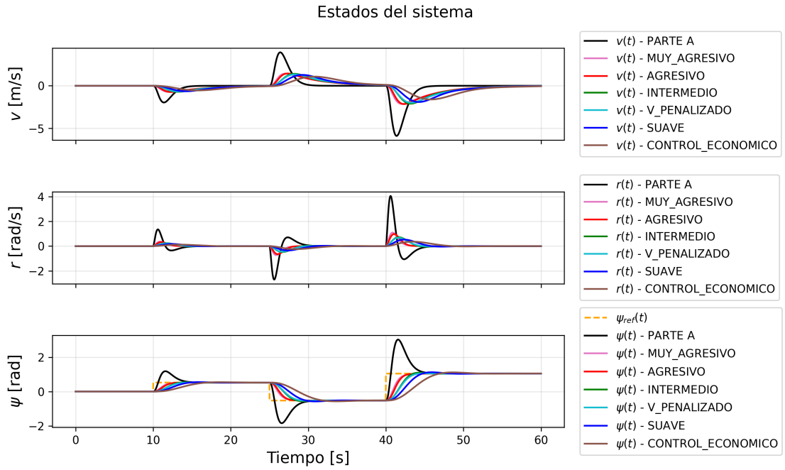
Figura 11: Comparación de estados entre Parte A y los controladores LQI.
