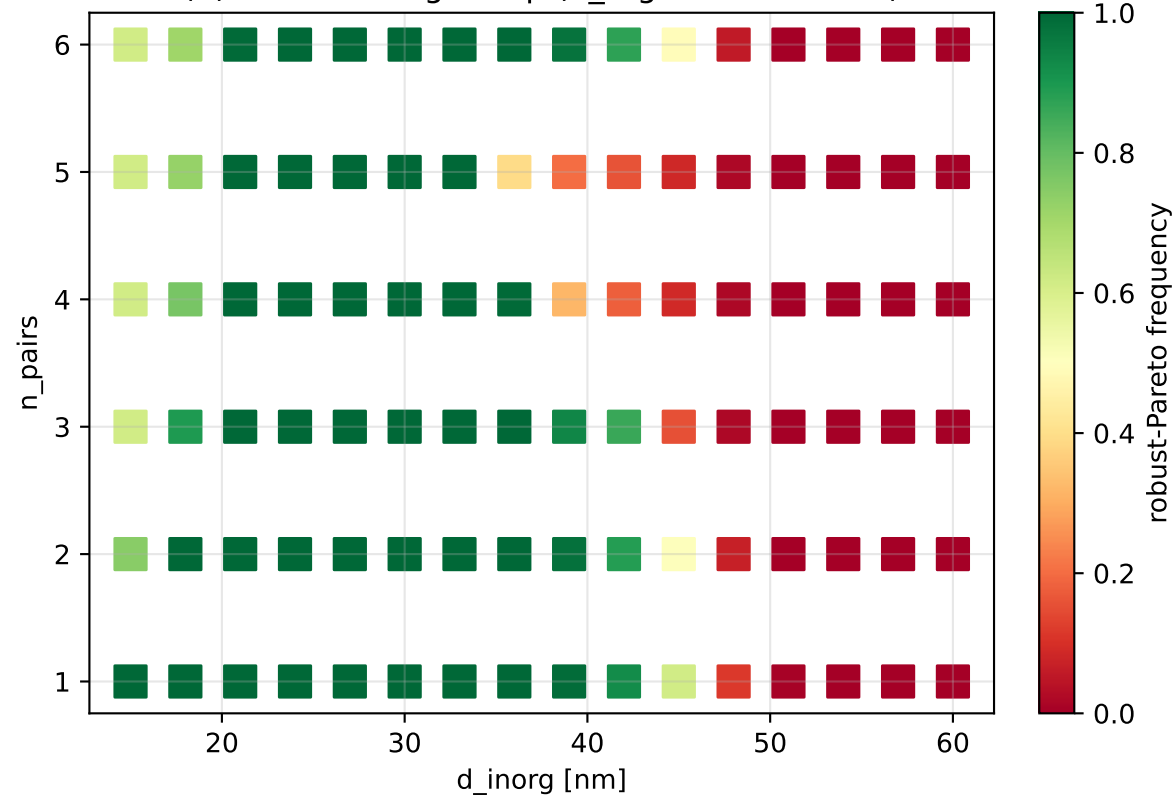
(d) Robust design map (d_org=100 nm slice)
