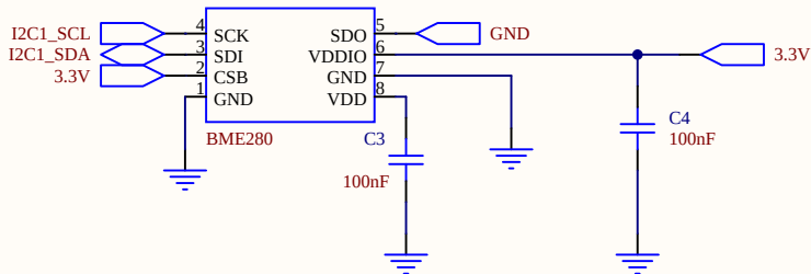
BME280
