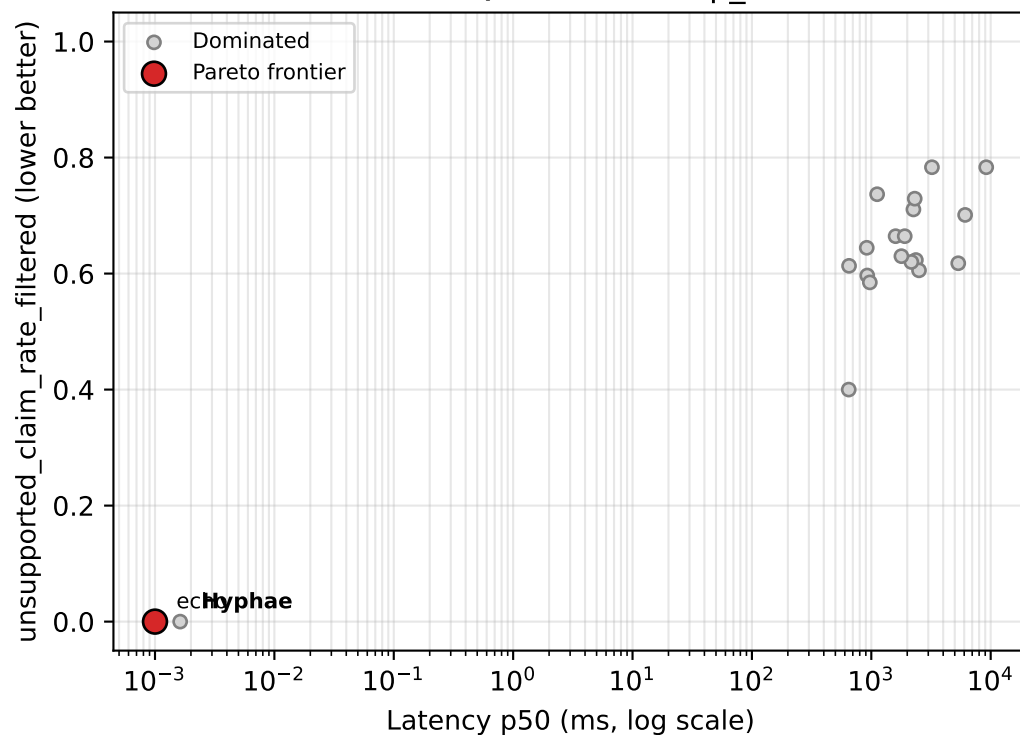
TriviaQA-150 -- unsup_f
