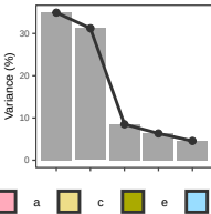
PCA Scree
