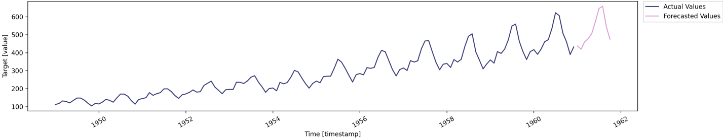
intrusion_attempts_20250109_015542: Forecasted vs Actual Values
