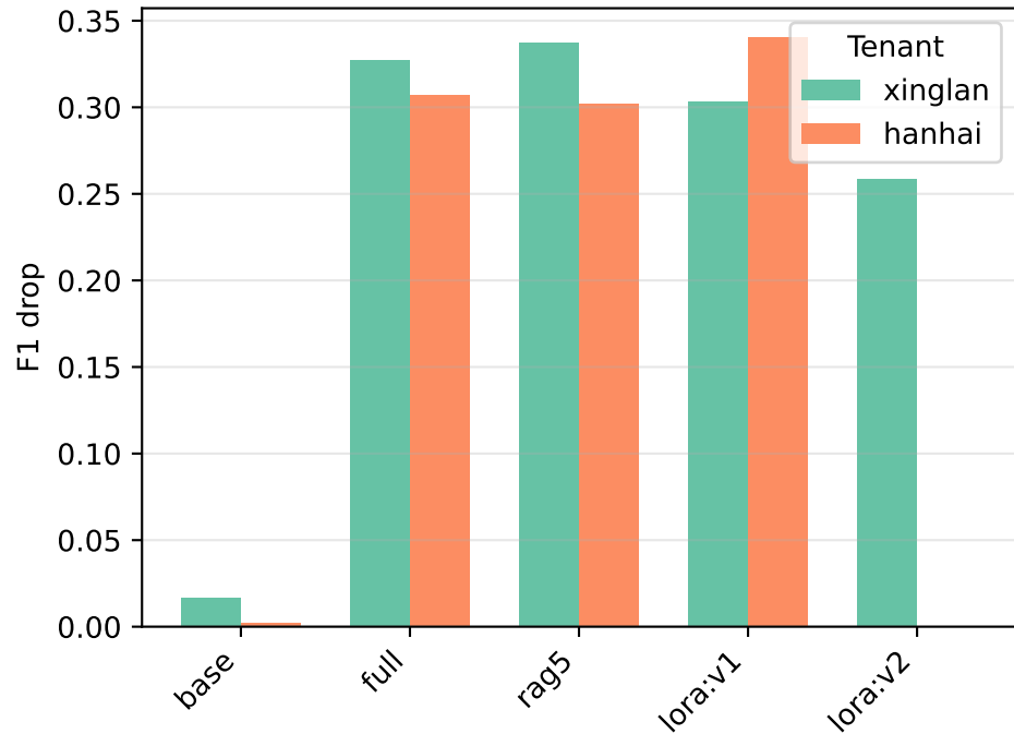
Own - Cross F1 drop
