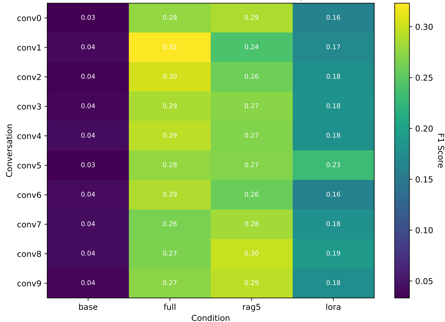
LoCoMo: Per-Conversation F1 Heatmap
