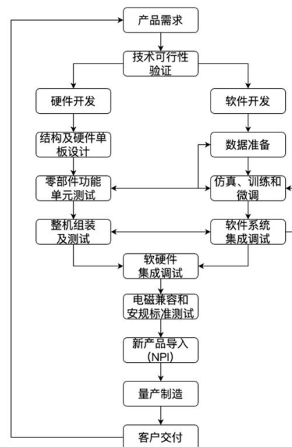
人形机器人研发参考流程
