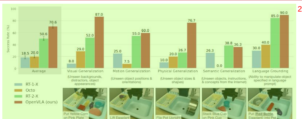
图表 34: Open VLA 模型在多项任务测评中相较于前代模型取得了更好的效果 1
