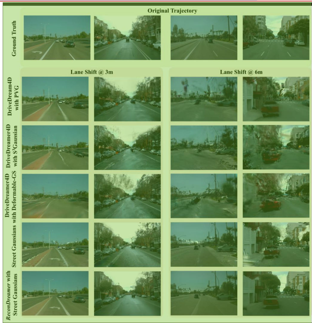
图表 19：理想 Recon Dreamer 模型长距离街景生成效果与传统方法的比较 1
