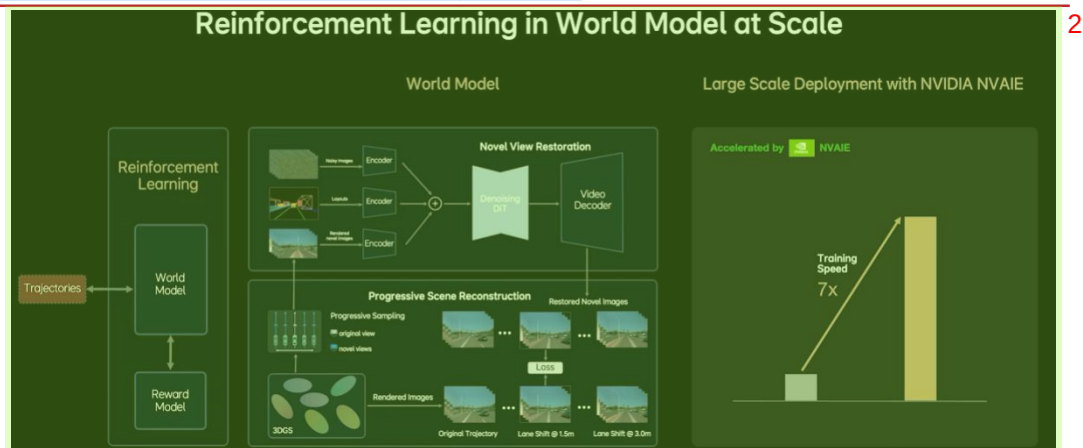
图表 26：理想 Mind VLA 后训练环节世界模型框架 1
