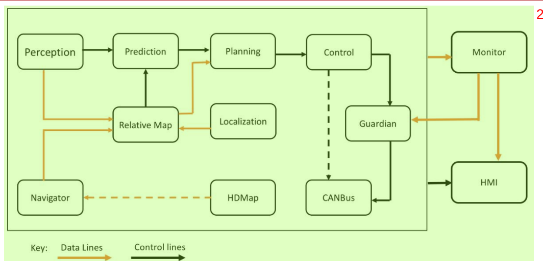
图表 1：百度 Apollo 算法架构具备典型感知、预测、规划、控制模块化特征 1
