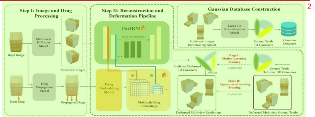
图表 31: PartRM 模型框架，通过观察预测形变与真实形变的差值进行隐式学习 1
