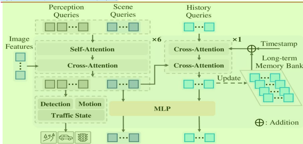
图表 11：小米 QT-Former 模型架构 2
