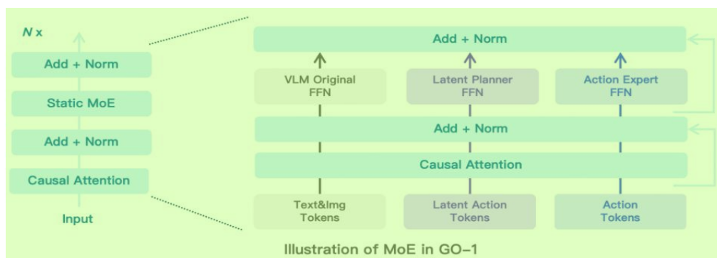
图表 39：GO-1 模型中的 MOE 层，包含 VLM、Latent Planner、Action Expert 三个核心组件 7
