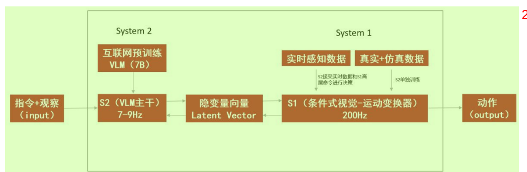
图表 35: Helix 模型架构 1
