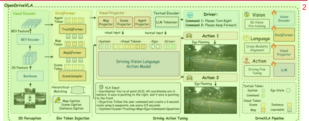
图表 22: Open Drive VLA 模型架构 1
