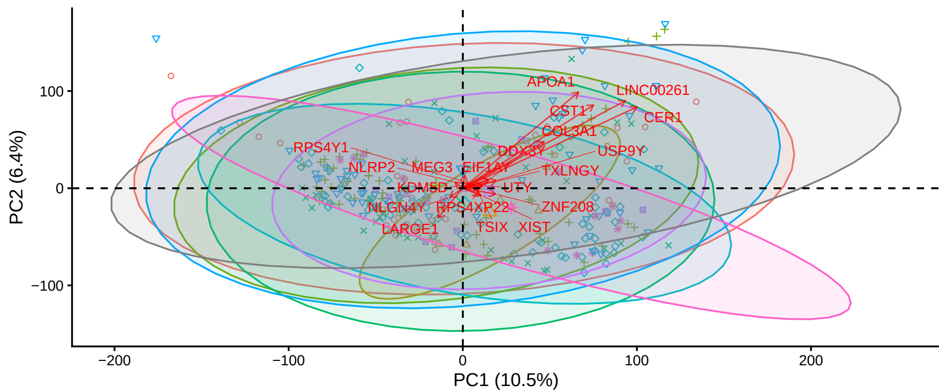
PCA – Biplot
