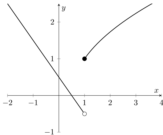
Slika 6.2: Graf funkcije iz zadatka 280
