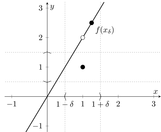
(b) Prekid funkcije iz zadatka 276 u 1
