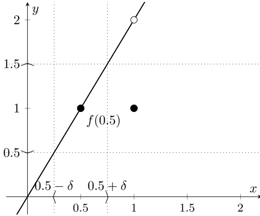
(a) Neprekidnost funkcije iz zadatka 276 u \frac{1}{2}
