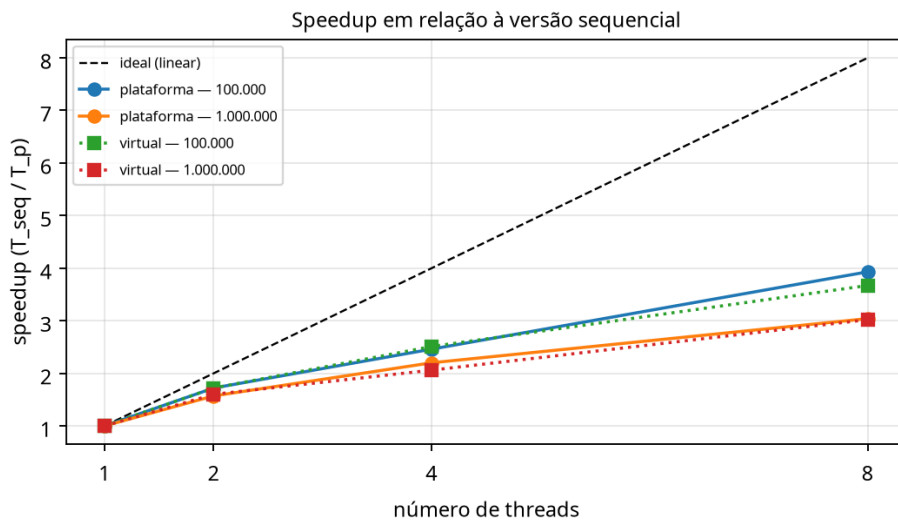
Figura 2 — Speedup \times número de threads (linha tracejada = speedup ideal).
