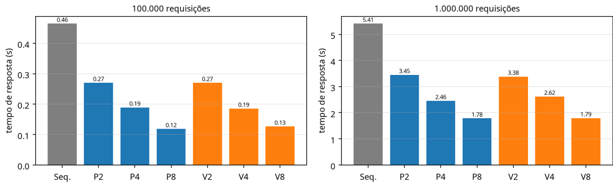
Figura 1 — Tempo de resposta do endpoint por versão e tamanho de entrada.
