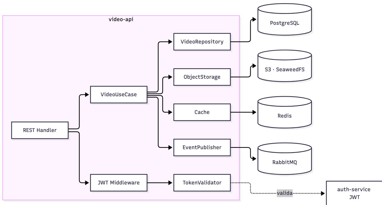
Nível 3 — Componente (video-api)
