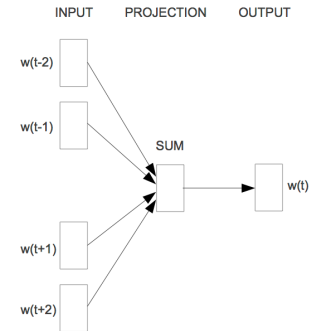
CBOW
