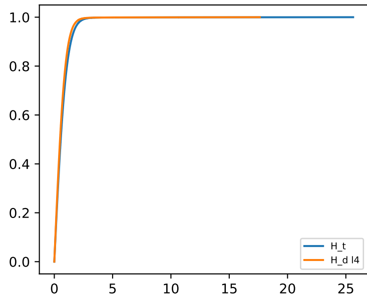
ECDF |x|
