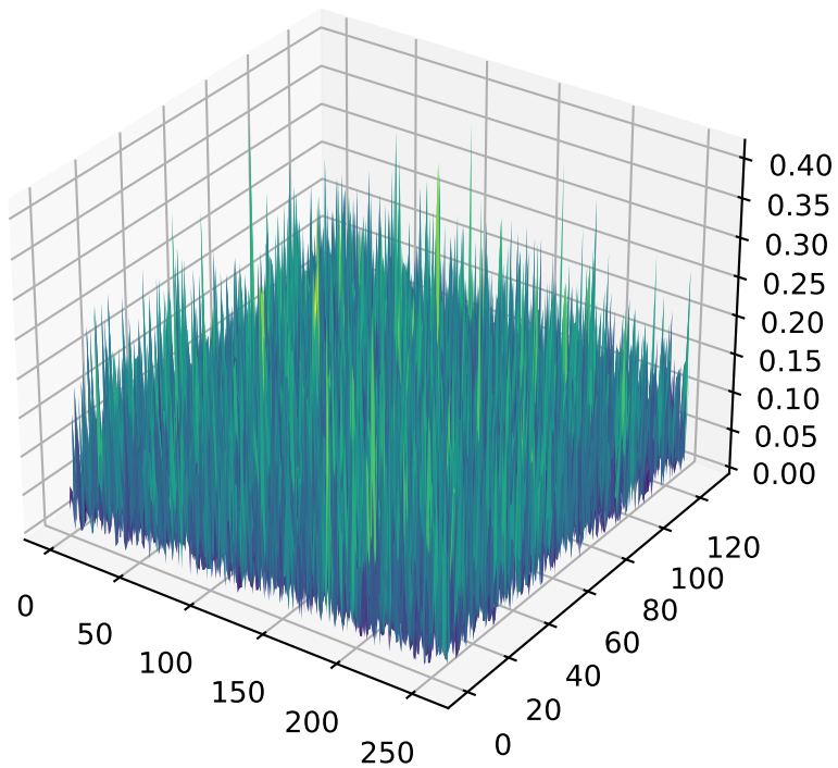
layer0 W_k_proj original
