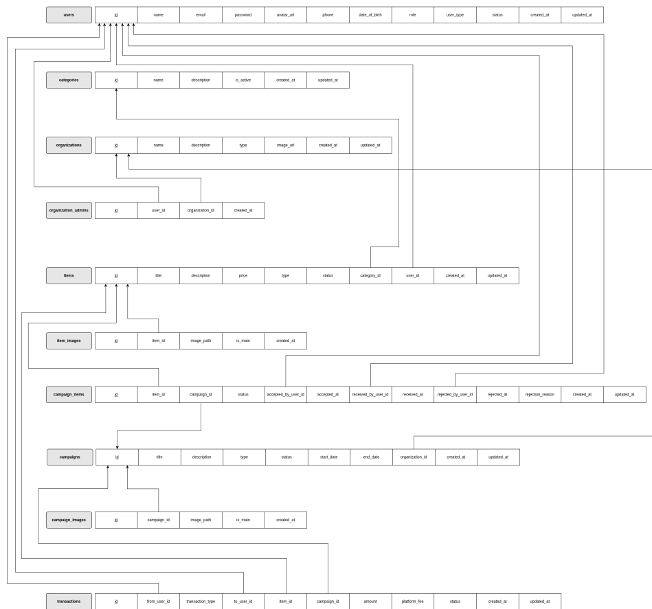
Hình 5.2: Relational Diagram
