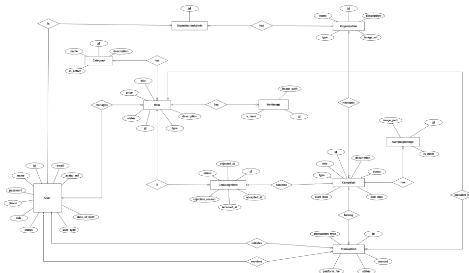
Hình 5.1: E-R Diagram
