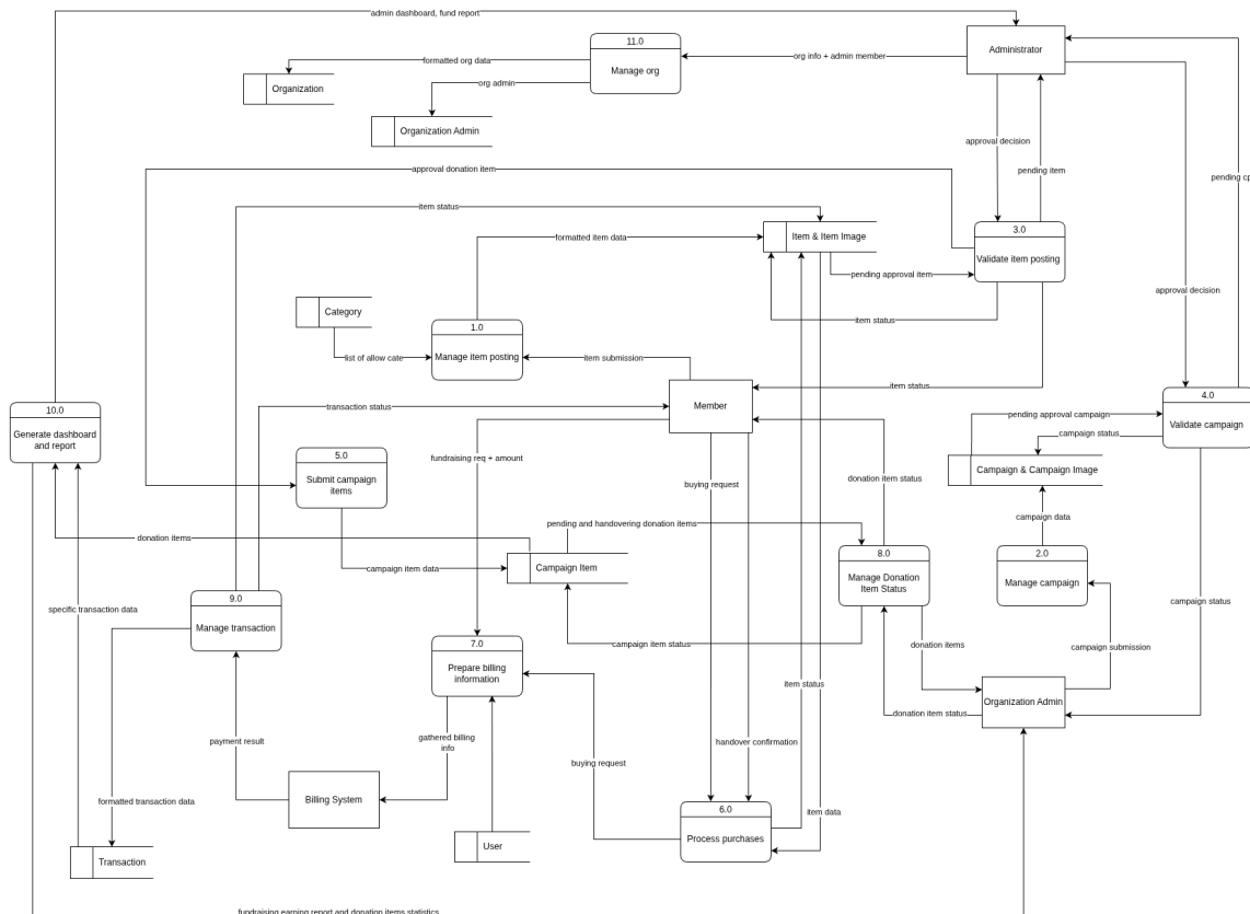
Hình 4.1. DFD Level 0
