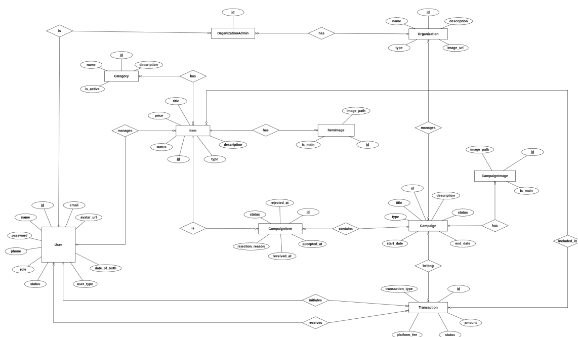
Hình 5.1. E-R Diagram
