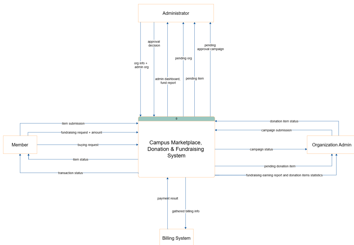
Hình 3.1. Context Diagram
