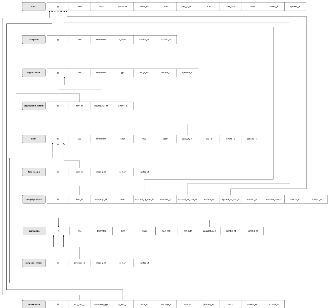
Hình 5.2. Relational Diagram
