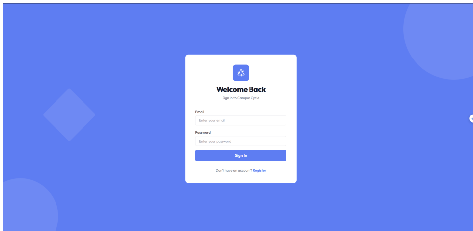
Hình 6.1: Login Page
