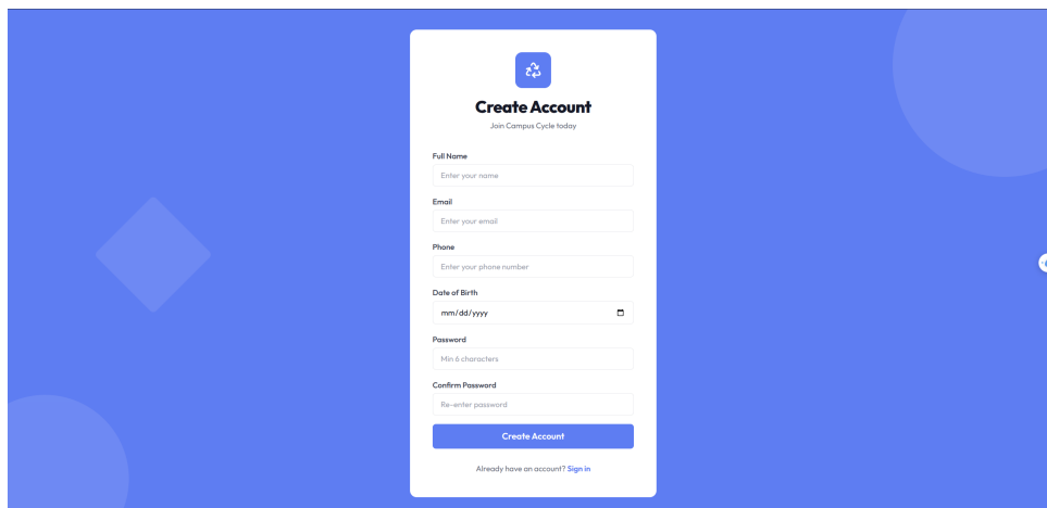
Hình 6.2: Register Page
