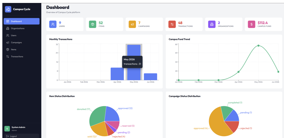
Hình 6.21: Admin Dashboard
