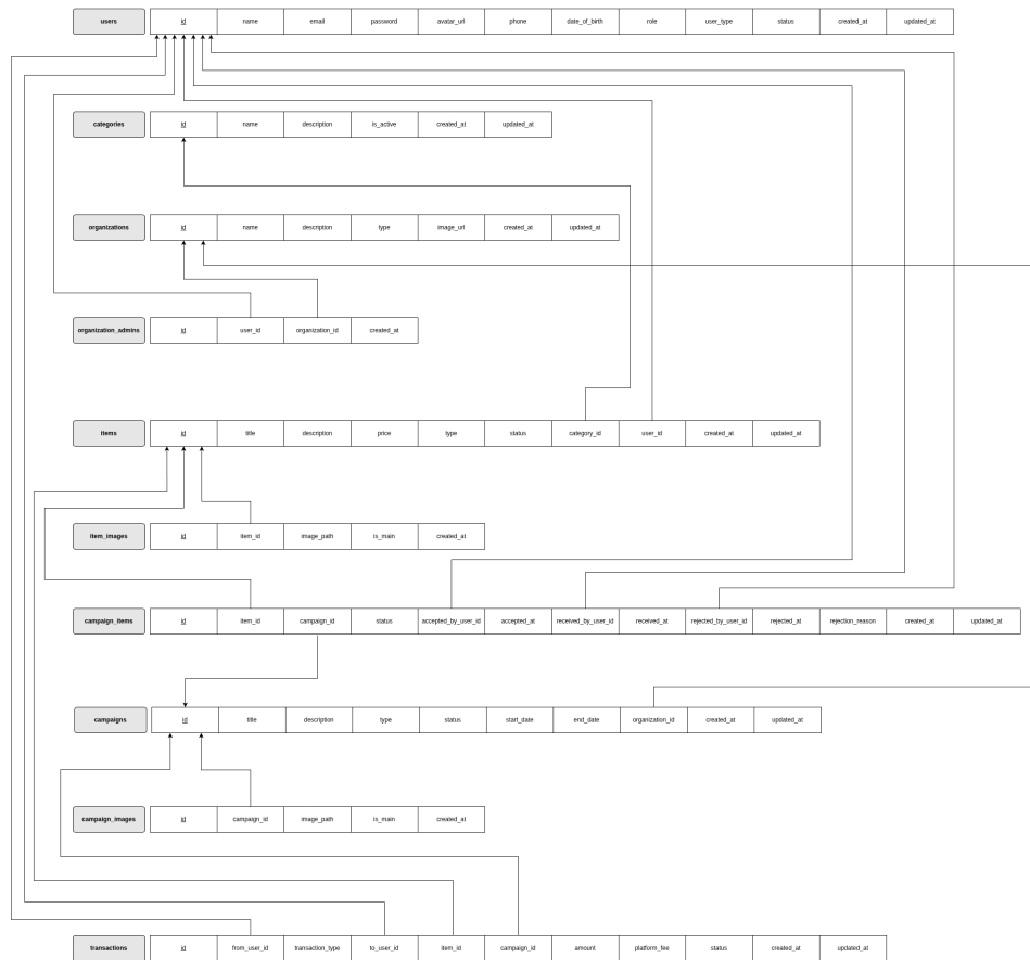
Hình 5.2: Relational Diagram
