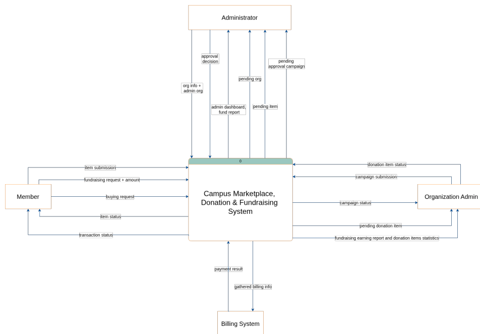
Hình 3.1: Context Diagram
