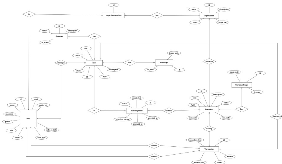
Hình 5.1: E-R Diagram
