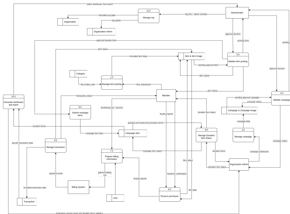
Hình 4.1: DFD Level 0
