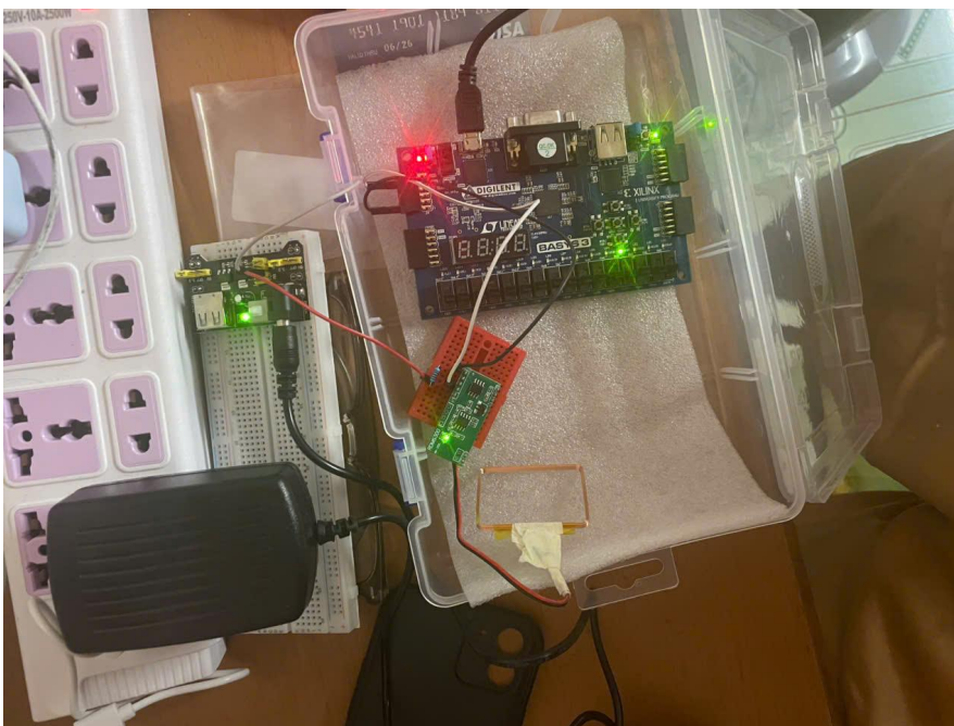
Hình 3: Thiết lập thực nghiệm phần cứng thực tế giữa FPGA Basys 3, Module nguồn MB102 5V và Đầu đọc RFID RDM6300
