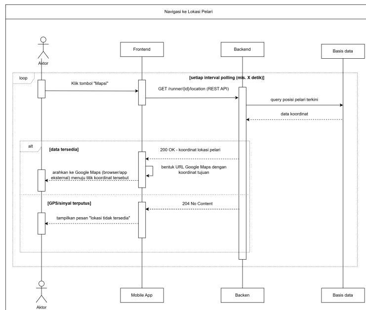
Gambar IV.11 Sequence Diagram Skenario Navigasi ke Lokasi Pelari
