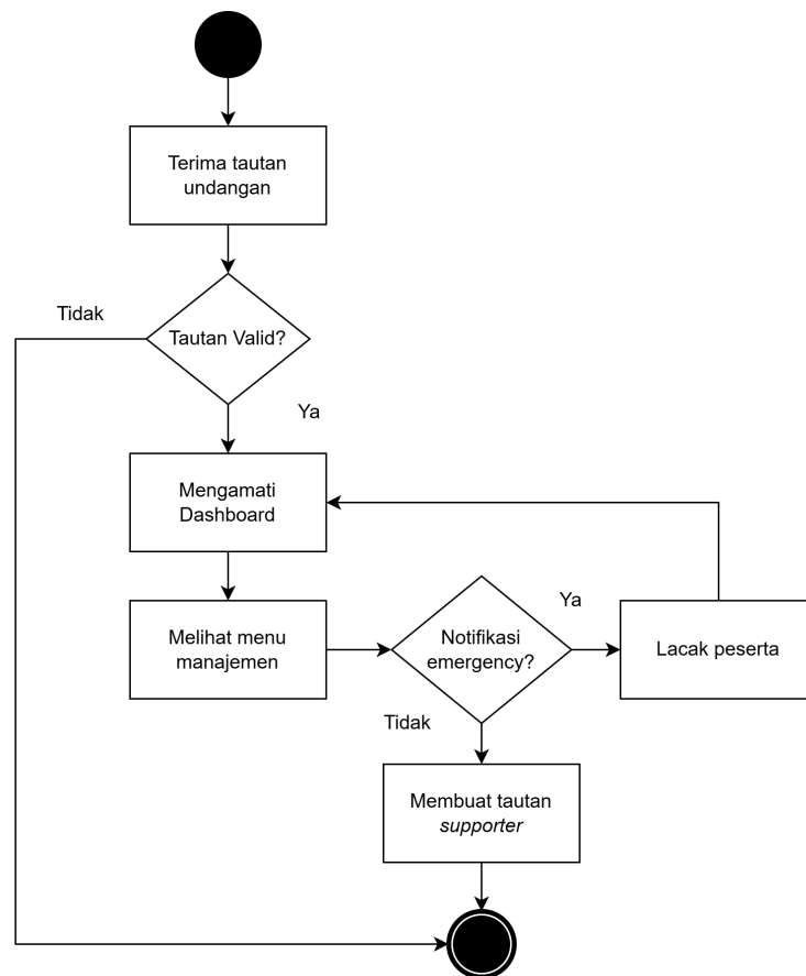
Gambar IV.14 User Flow Ketua Tim
