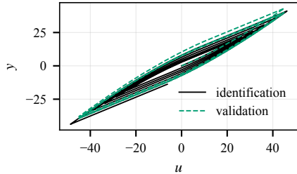
E3: Bouc–Wen hysteresis
