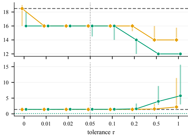
E3: Bouc–Wen hysteresis
