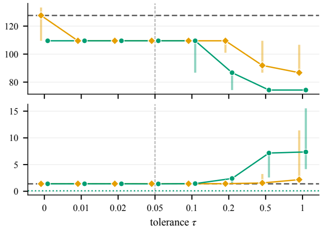
E3: Bouc–Wen hysteresis
