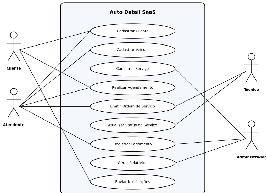
Figura 1 – Diagrama de Casos de Uso do Auto Detail SaaS. Fonte: elaborado pelo autor (2026).
