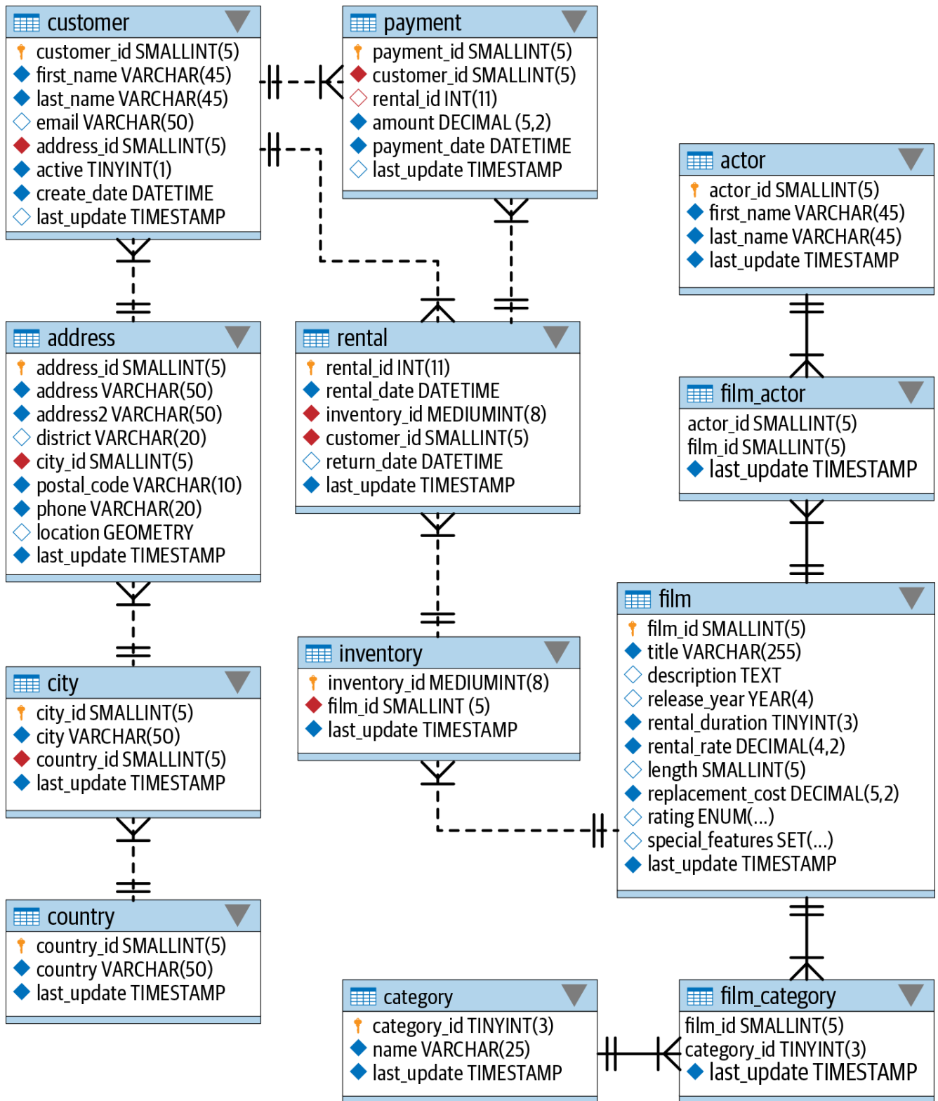
Figure A-1. ER diagram
