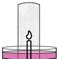
Condição inicial Vela acesa e solução rosada
