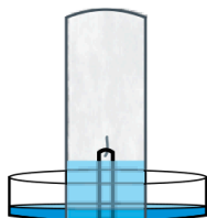
Condição final Vela apagada e solução incolor
