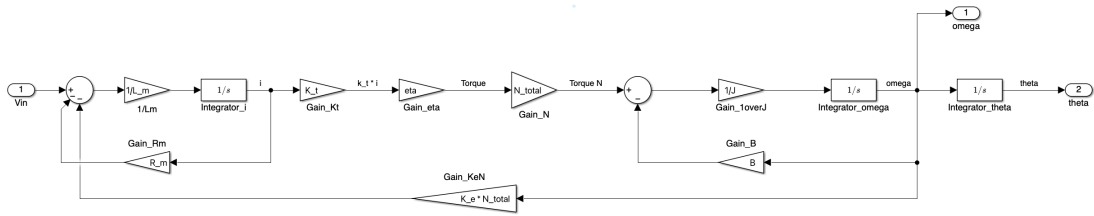
รูปที่ 13: Block Diagram ของระบบมอเตอร์กระแสตรงพร้อมชุดทดรอบใน Simulink
