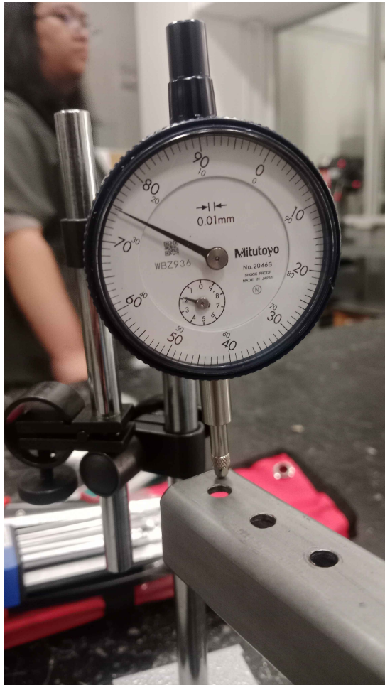
(a) ตำแหน่งที่ใช้ Dial Gauge บนโครงสร้างชิ้นงานจริง
