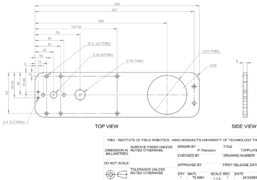
รูปที่ 46: Engineering Drawing: Top plate
