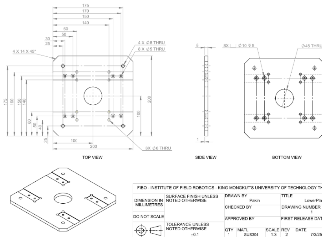
รูปที่ 45: Engineering Drawing: Lower plate
