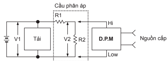
(Hình 2) Đo điện áp cao hơn 300VDC của điện áp đo
