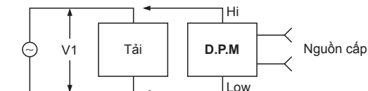
(Hình 3) Đo điện áp thấp hơn 400VAC của điện áp đo (V1)
