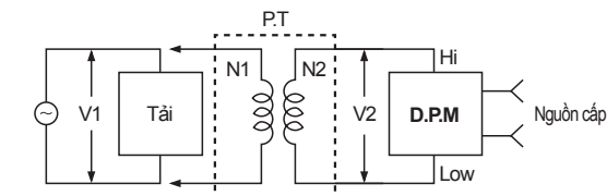
(Hình 4) Đo điện áp cao hơn 400VAC của điện áp đo (V1)
