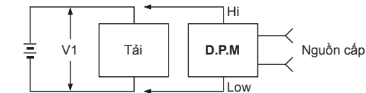
(Hình 1) Đo điện áp thấp hơn 300VDC của điện áp đo (V1)
