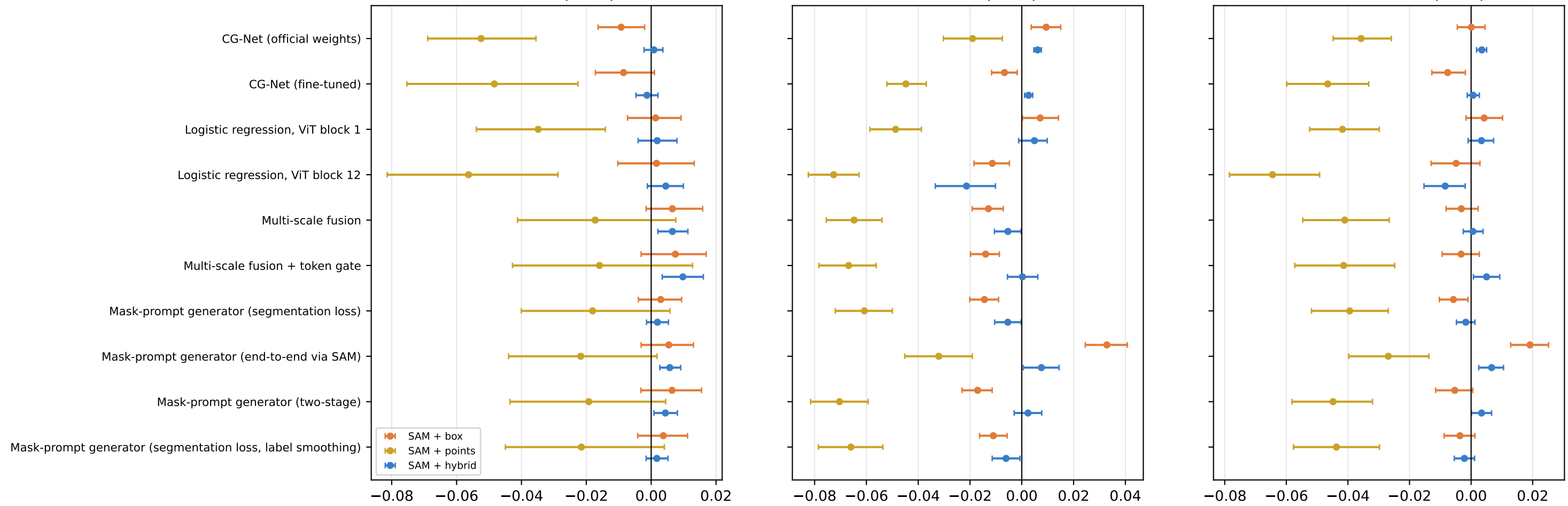
TC IoU: SAM minus prompter mask
