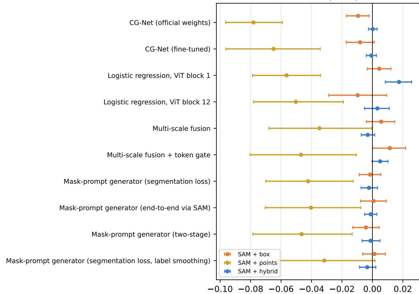
TC IoU: SAM minus prompter mask
