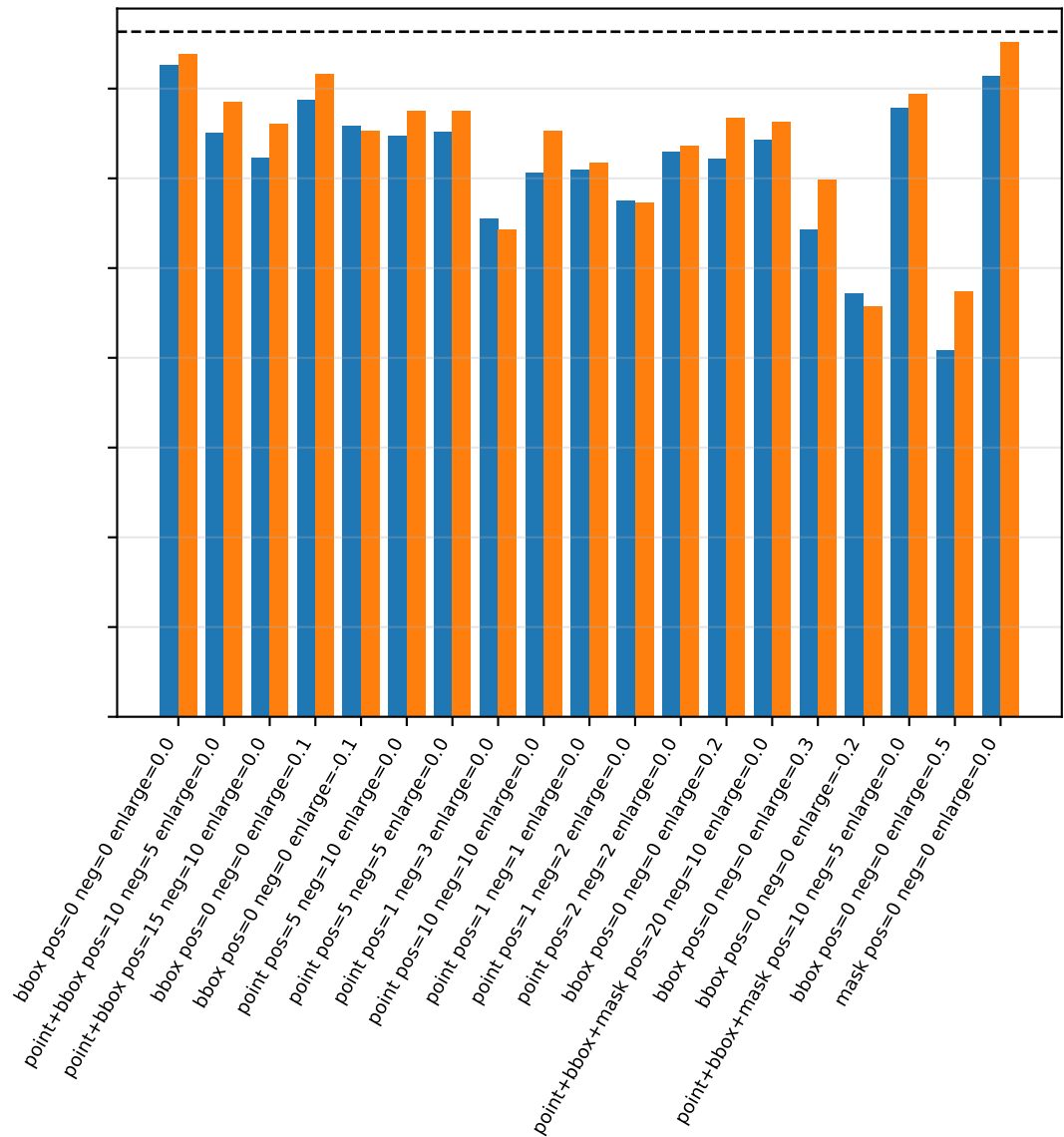
AR IoU
