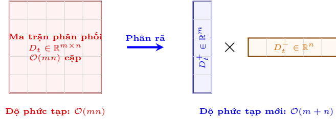
Hình 9: Bản chất đột phá của BipartiteRankBoost: Phân rã ma trận phân phối cặp toàn cục D_t(i, j) thành tích của hai vector phân phối biên D_t^+(i) và D_t^-(j) . Chuyển hóa độ phức tạp tính toán và lưu trữ từ bậc hai \mathcal{O}(mn) sang tuyến tính \mathcal{O}(m+n) .
