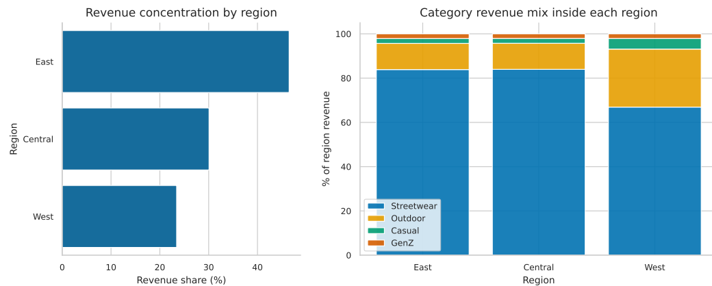
Figure 7: Revenue concentration và category mix theo vùng. Sources: geography, orders, order_items, products.
