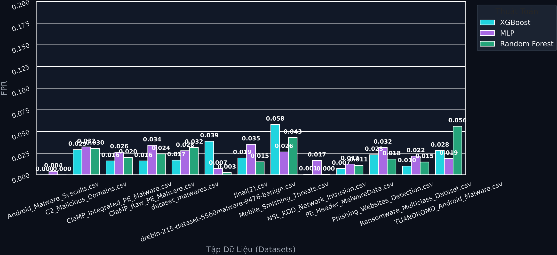
So sánh FPR - False Positive Rate (Tỷ lệ báo động giả - Càng thấp càng an toàn)
