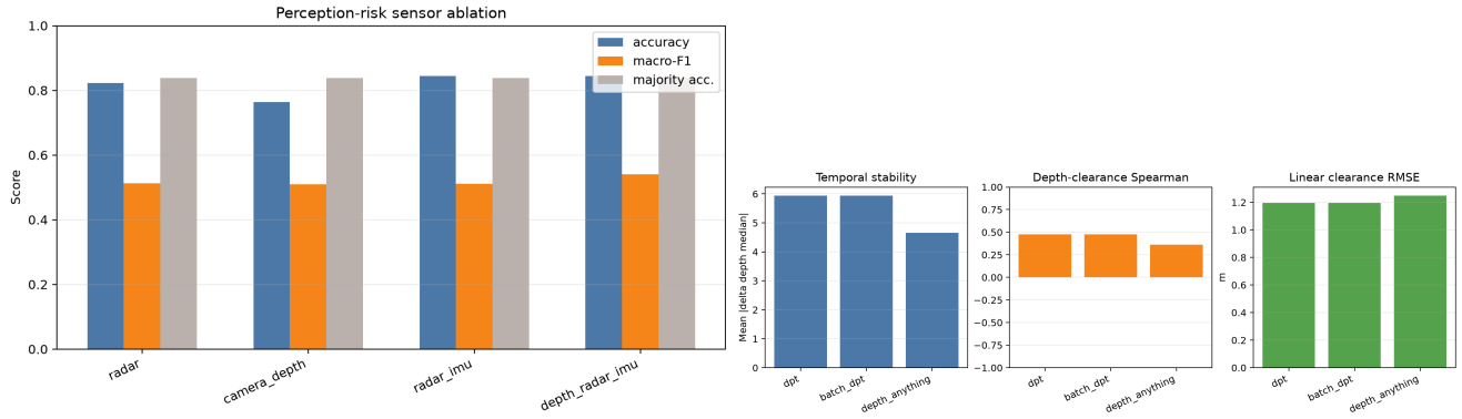
Figure 3: Ablation feature cho DPT-Hybrid/MiDaS và phân tích stability/calibration giữa relative depth, radar feature và clearance.
