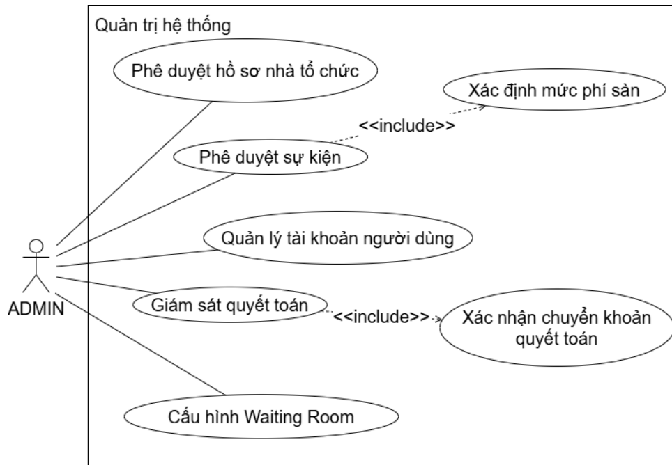
Hình 2.4: Biểu đồ use case phân rã nhóm chức năng quản trị hệ thống
