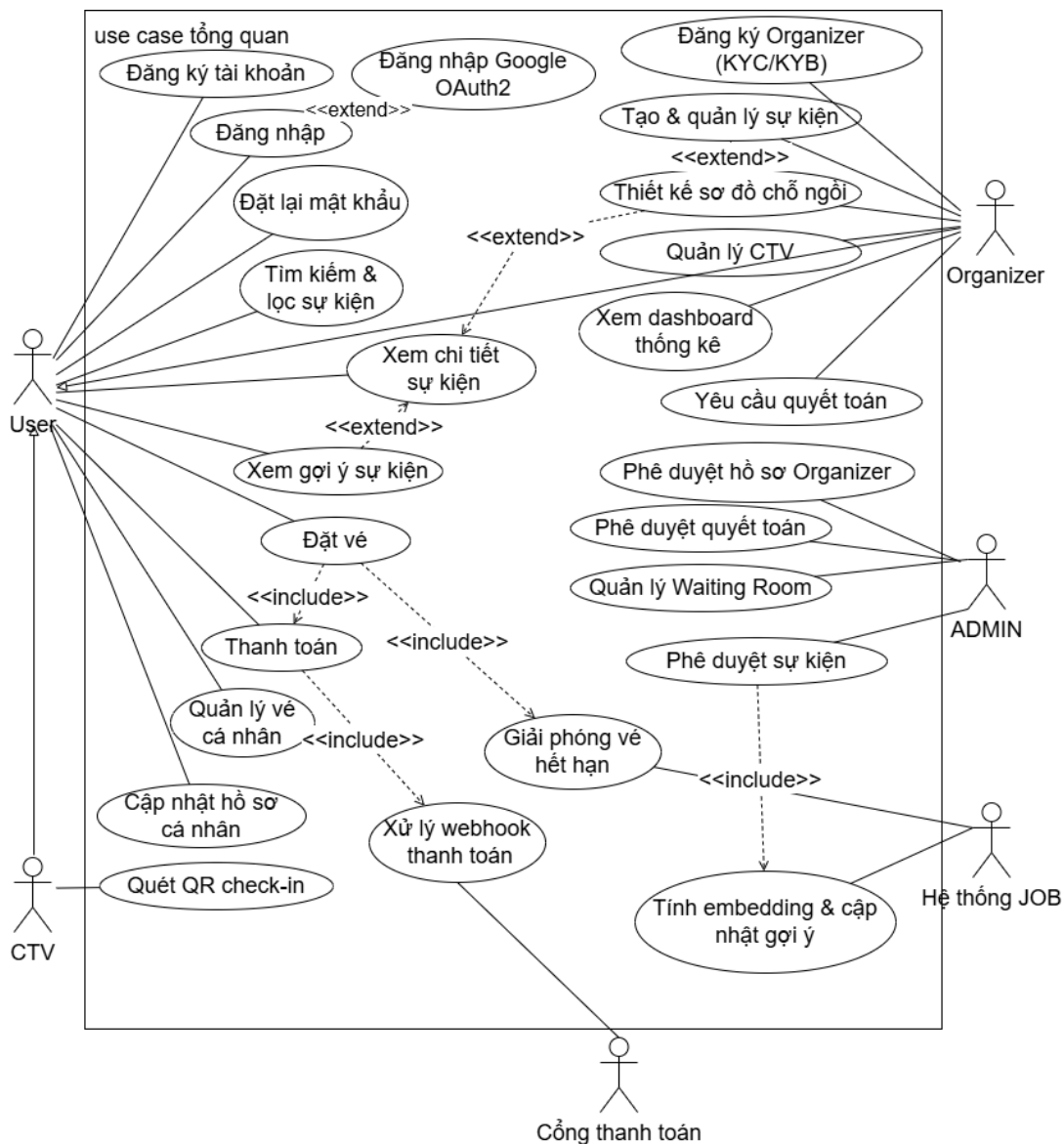
Hình 2.1: Biểu đồ use case tổng quát của hệ thống
