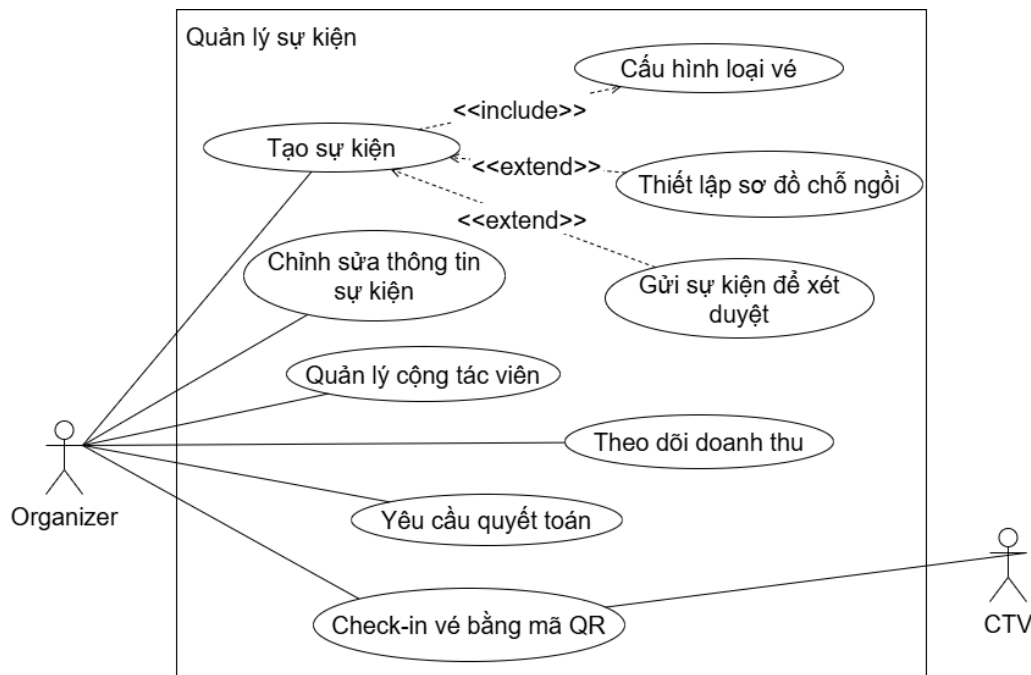
Hình 2.3: Biểu đồ use case phân rã nhóm chức năng quản lý sự kiện
