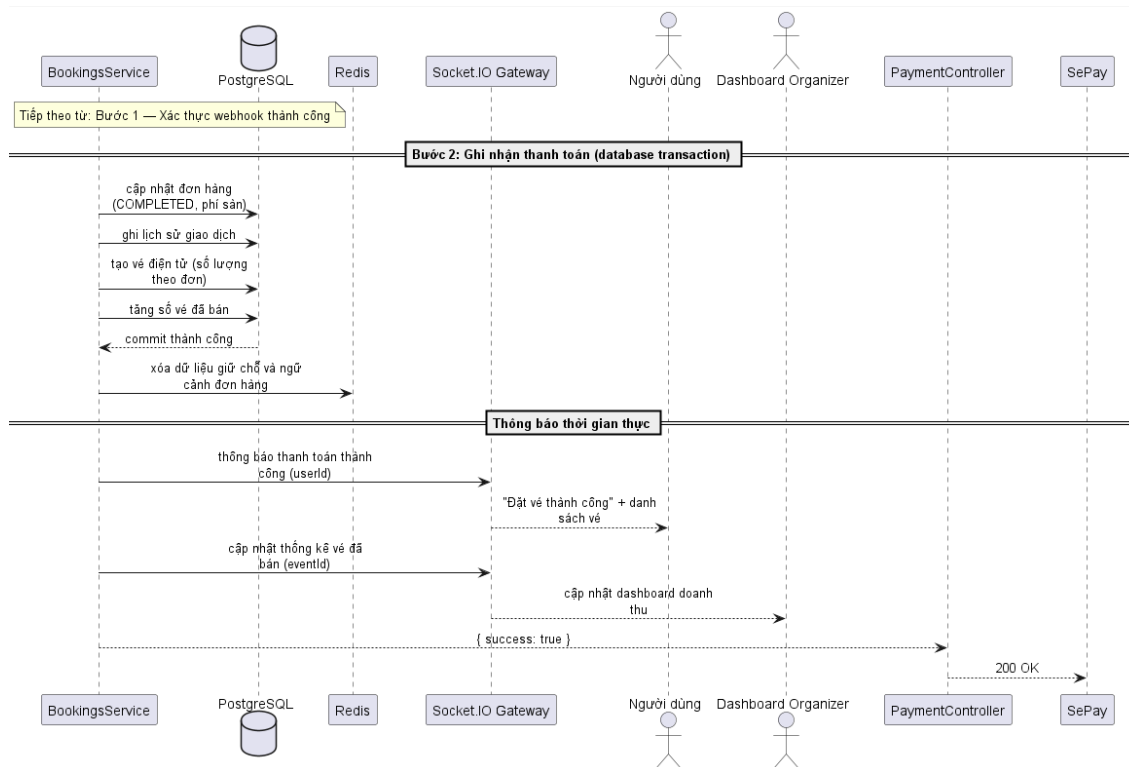
Hình 4.10: Biểu đồ trình tự luồng xác nhận thanh toán qua webhook SePay — Bước 2: Ghi nhận thanh toán và thông báo thời gian thực
