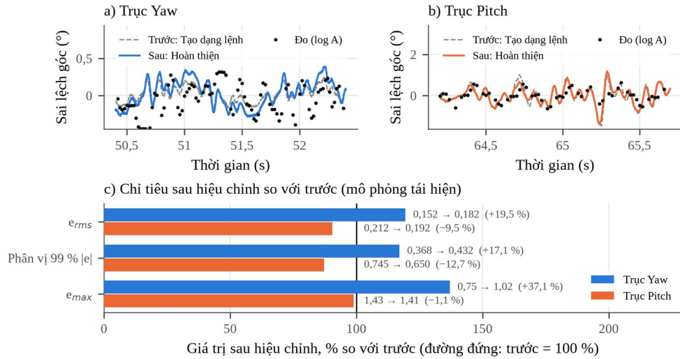
Hình 3.20. Trước và sau hoàn thiện lịch truyền RS485: mô phỏng tái hiện và số đo log A
