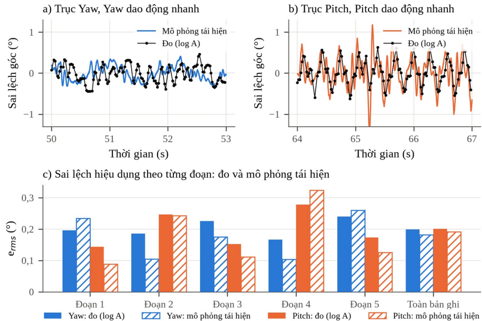
Hình 3.6. Kiểm chứng mô hình tái hiện với log A của cấu hình hoàn thiện
