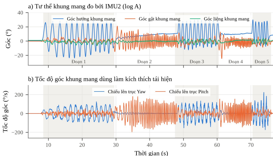
Hình 3.5. Bài thử tham chiếu: chuyển động khung mang ghi trong log A
