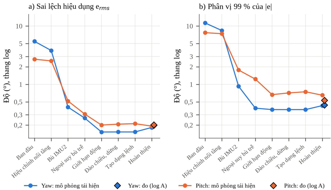
Hình 3.22. Chỉ tiêu sai lệch qua các bước hiệu chỉnh trên bài thử tham chiếu
