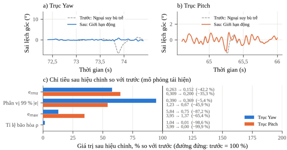
Hình 3.14. Trước và sau bổ sung giới hạn lệnh theo trạng thái động (mô phỏng tái hiện)
