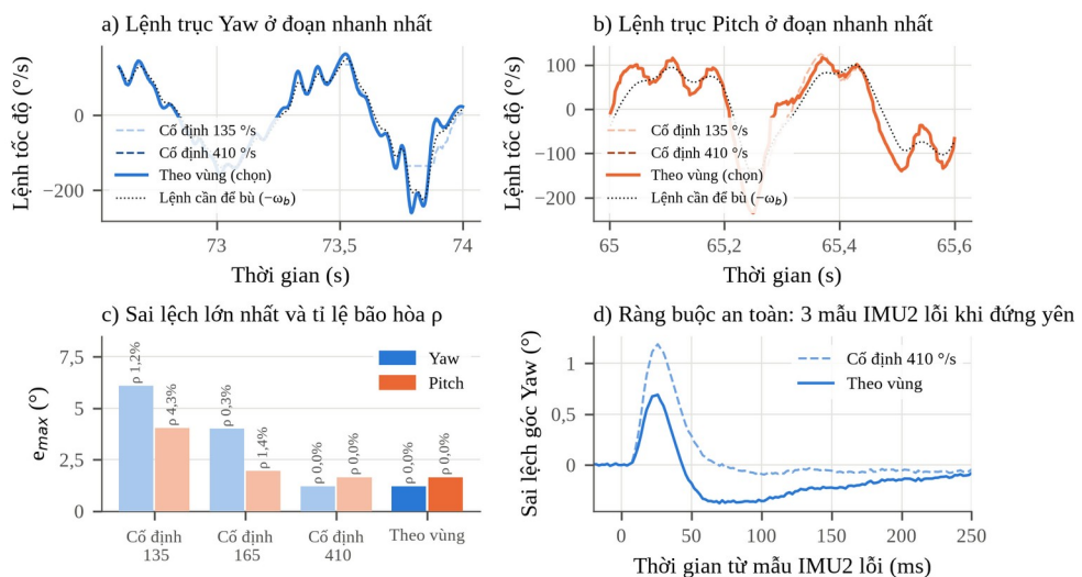
Hình 3.13. Mô phỏng khảo sát luật giới hạn lệnh
