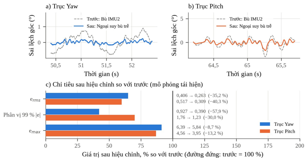
Hình 3.12. Trước và sau bổ sung ngoại suy bù trễ (mô phỏng tái hiện)
