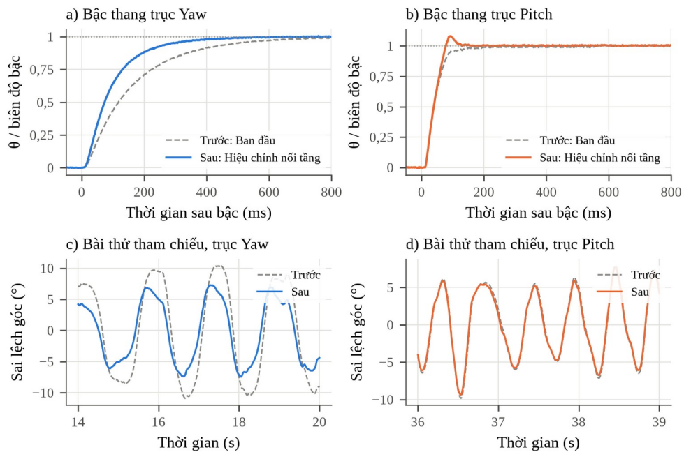
Hình 3.8. Trước và sau hiệu chỉnh bộ điều khiển nối tầng (mô phỏng tái hiện)
