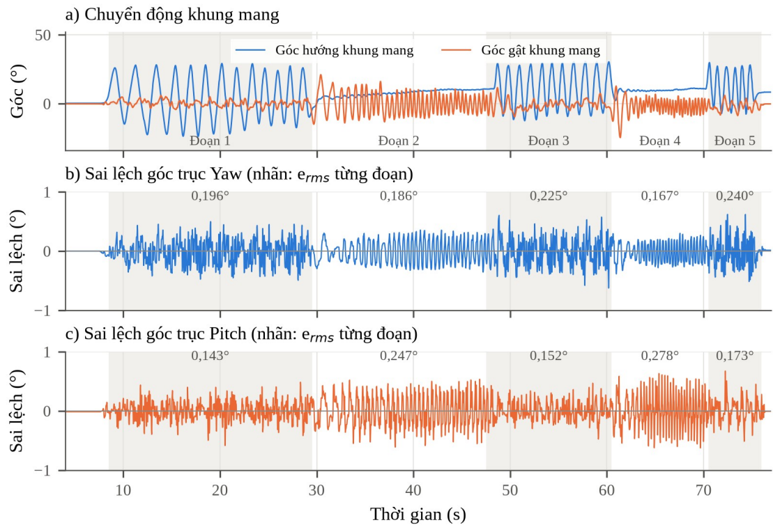
Hình 3.21. Kết quả đo cấu hình hoàn thiện trên bài thử tham chiếu (log A)
