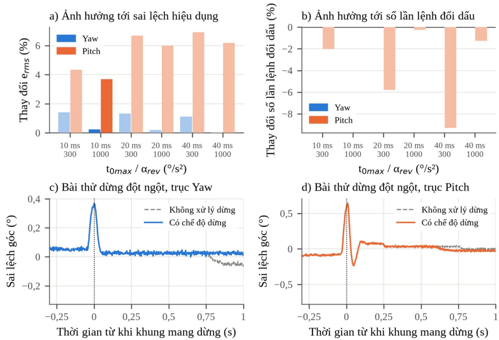
Hình 3.15. Mô phỏng khảo sát tham số xử lý đảo chiều và chế độ dừng
