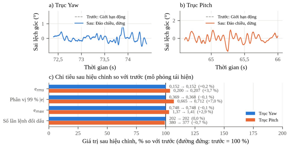
Hình 3.16. Trước và sau bổ sung xử lý đảo chiều và dừng (mô phỏng tái hiện)
