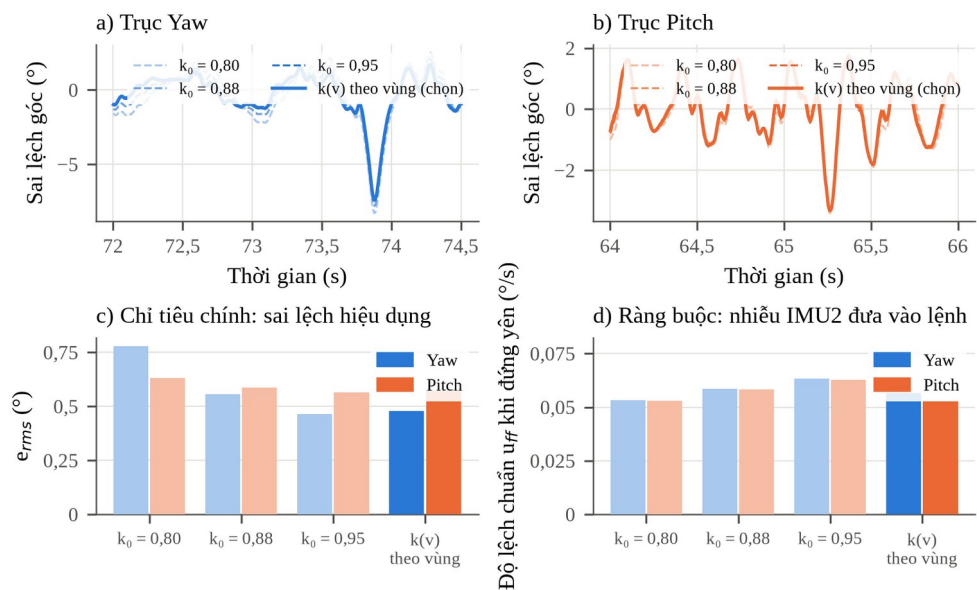
Hình 3.9. Mô phỏng khảo sát luật hệ số bù chuyển động khung mang
