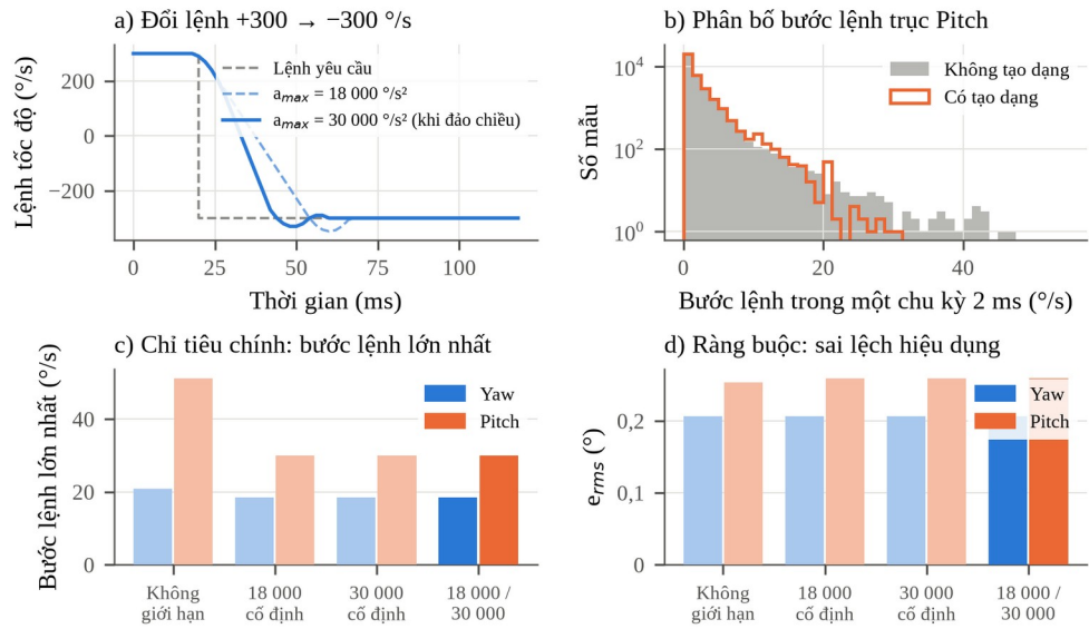
Hình 3.17. Mô phỏng khảo sát khâu tạo dạng lệnh
