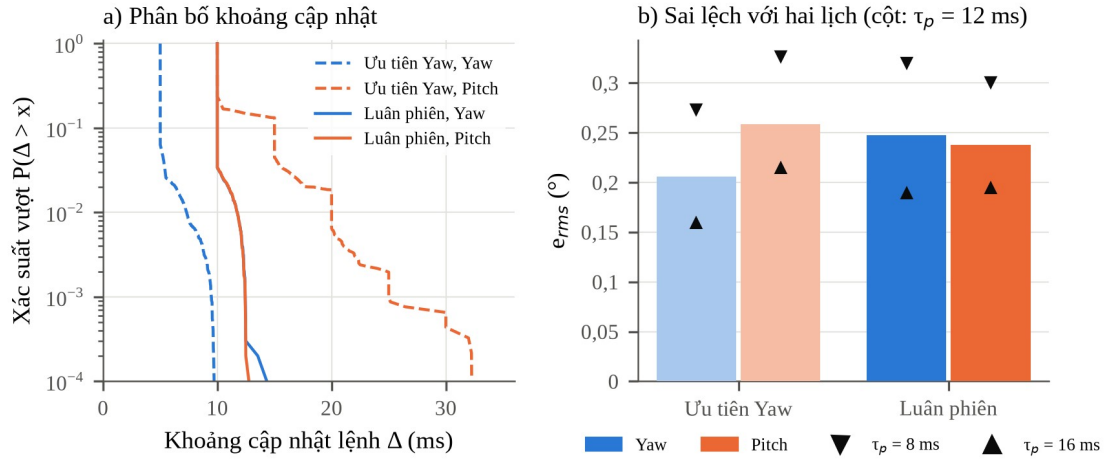
Hình 3.19. Mô phỏng khảo sát hai phương án lập lịch RS485
