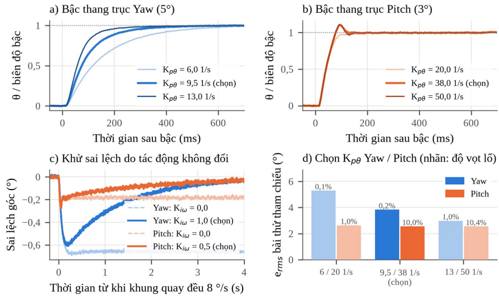
Hình 3.7. Mô phỏng khảo sát bộ hệ số nối tầng trên hai trục
