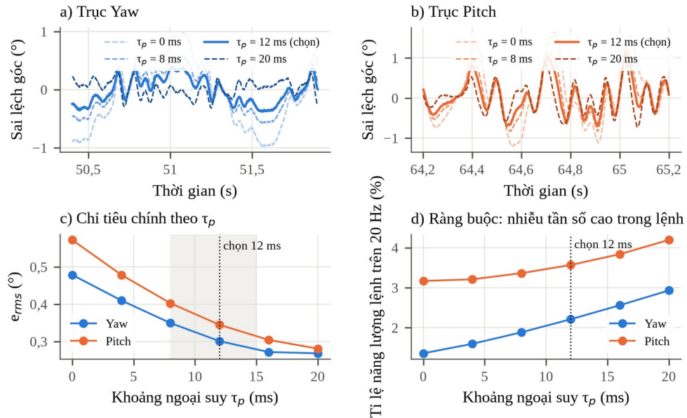
Hình 3.11. Mô phỏng khảo sát khoảng ngoại suy bù trễ
