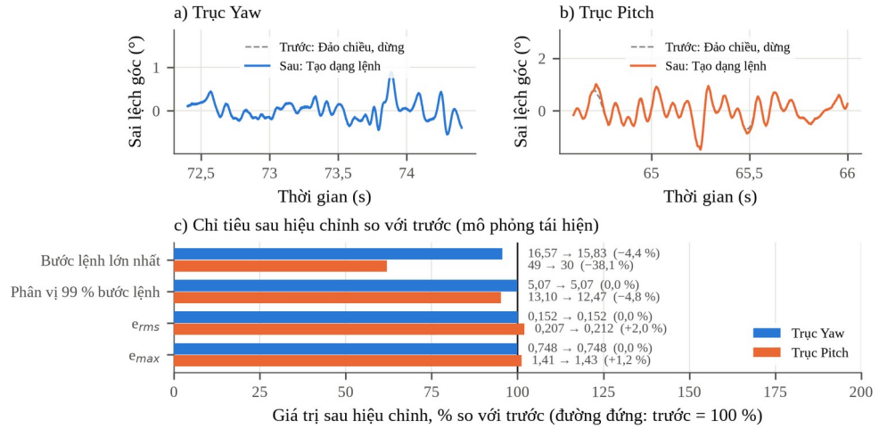
Hình 3.18. Trước và sau bổ sung khâu tạo dạng lệnh (mô phỏng tái hiện)
