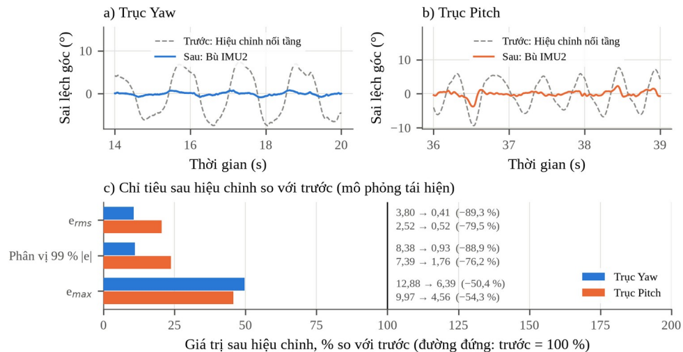
Hình 3.10. Trước và sau bổ sung bù chuyển động khung mang từ IMU2 (mô phỏng tái hiện)
