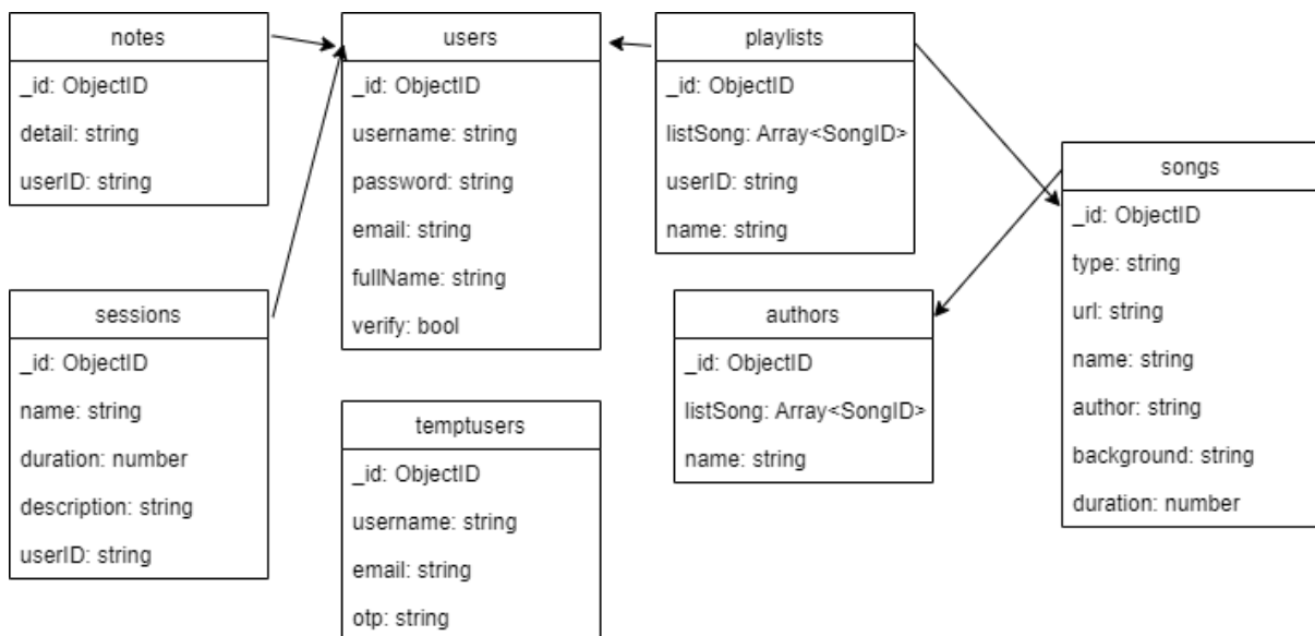
Hình 2.1 Sơ đồ thiết kế database
