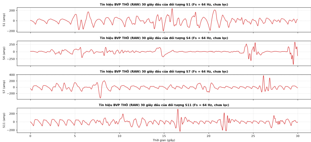
Hình 1: Dạng sóng BVP thô đại diện
