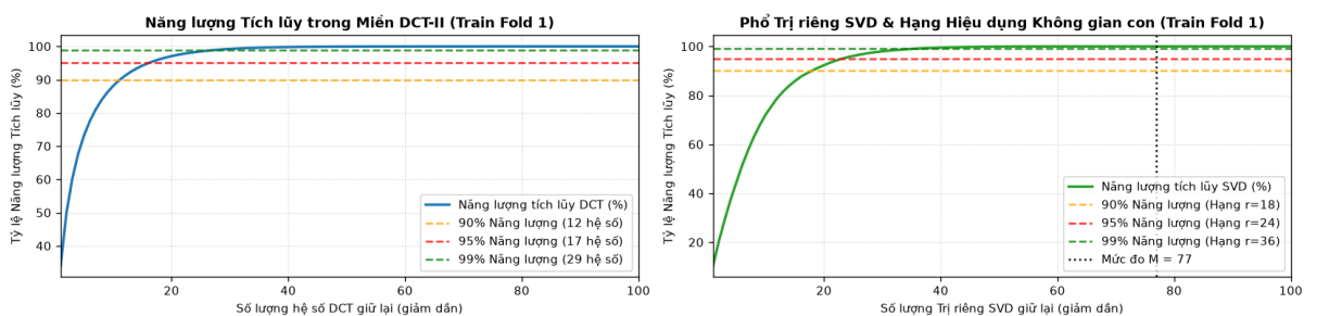
HÌNH 5: PHÂN TÍCH ĐỘ NÉN THUA DCT VÀ PHỔ TRỊ RIÊNG SVD TRÊN TẬP TRAIN (FOLD 1)
