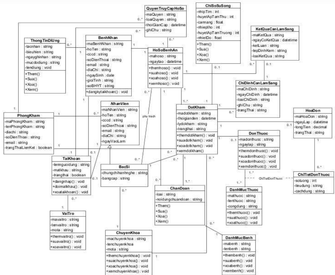
Hình 3.2 Sơ đồ Class hệ thống quản lý bệnh án liên phòng khám tư nhân
