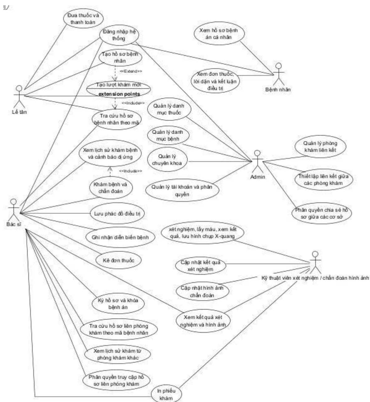
Hình 3.1 Sơ đồ Use Case hệ thống quản lý bệnh án liên phòng khám tư nhân
