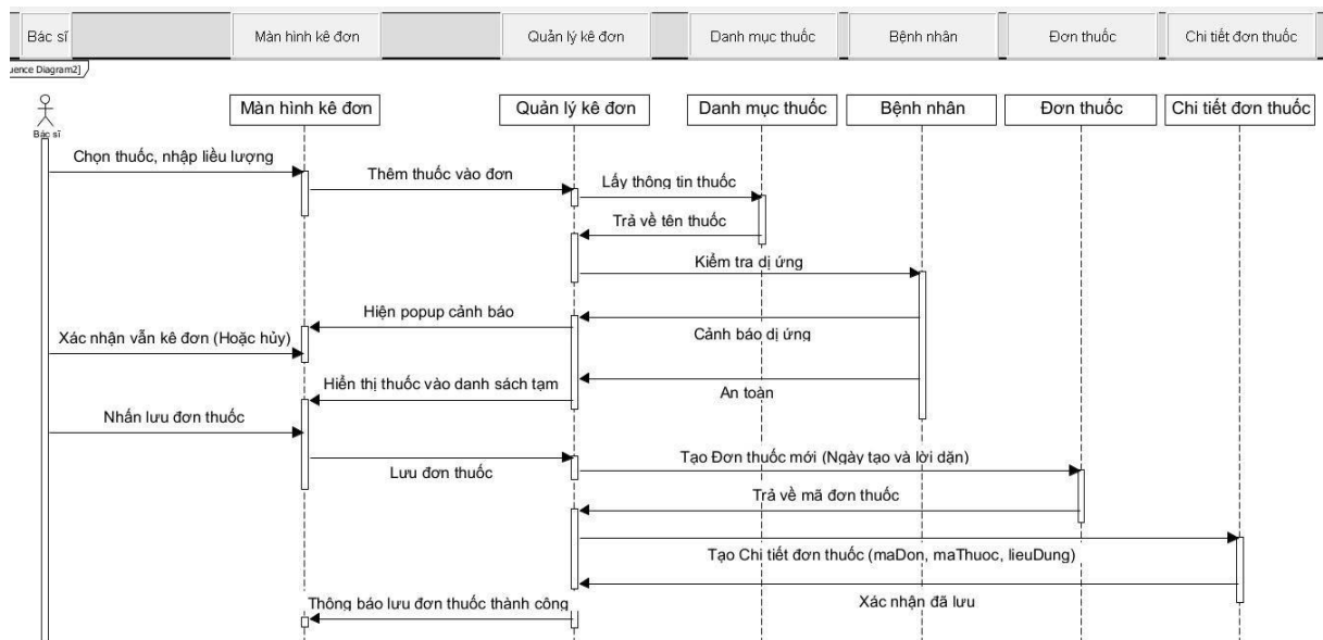
Hình 3.5 Đặc tả luồng tương tác quy trình kê đơn thuốc của Bác sĩ
