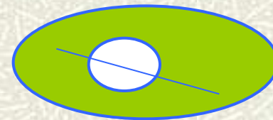
(c)非凸集
