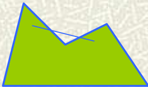
(a)非凸集
