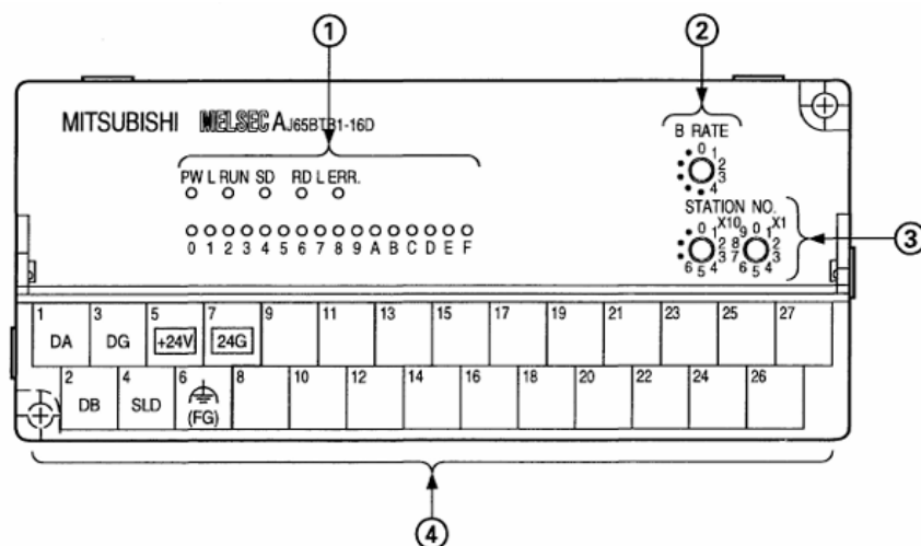
Hình 1.22. Phần cứng Remote IO
