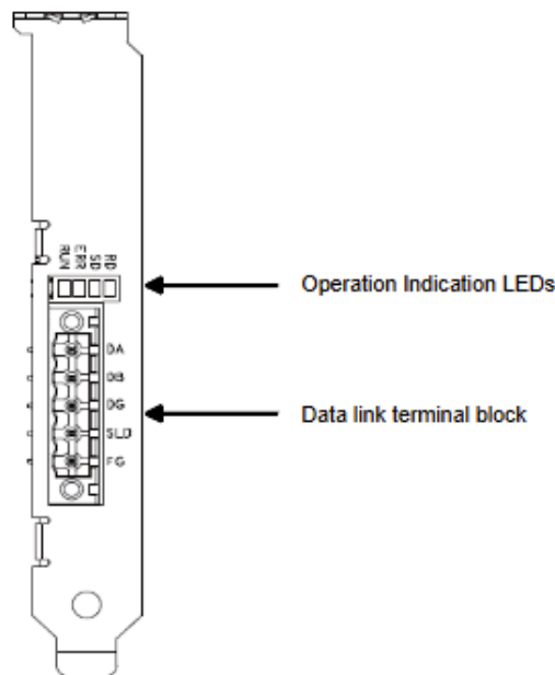
Hình 1.26. Board CCS-PCIE
