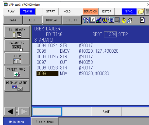
Hình 1.29. Ladder Program
