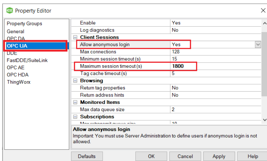
Hình 1.17. Cấu hình Project Kepware
