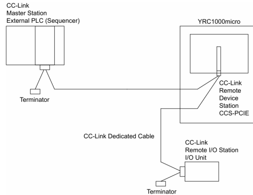
Hình 1.25. Kết nối CC-Link giữa Robot Yaskawa và PLC
