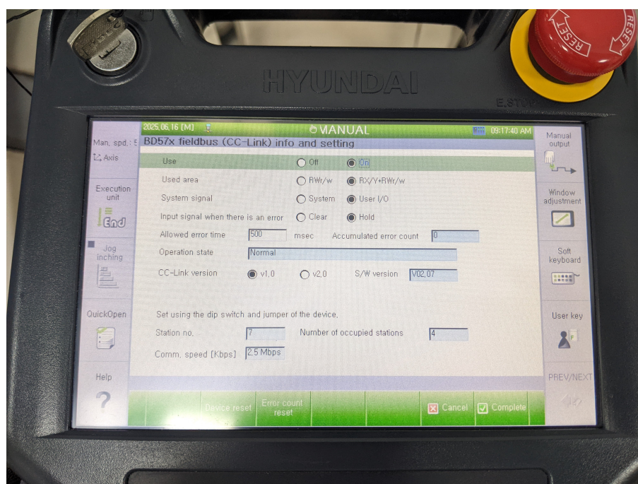
Hình 1.24. Thông tin thiết lập CC-Link
