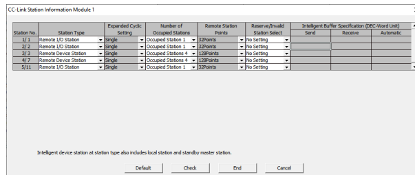
Hình 1.15. Master Station Setup
