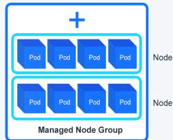
Cluster Autoscaler
