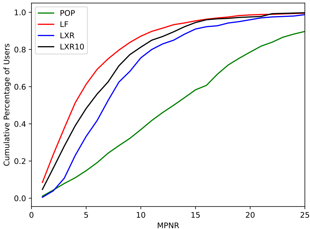
Recommender:MF, Dataset:Pinterest
