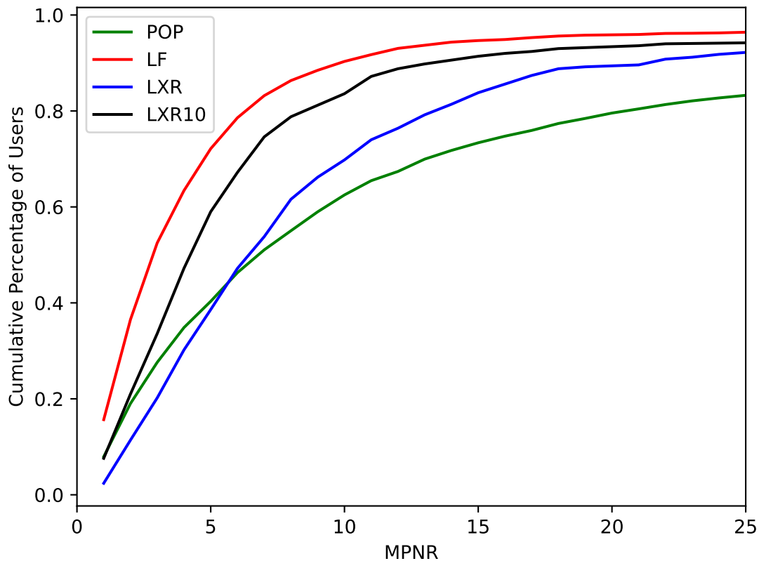
Recommender:MF, Dataset:Yahoo
